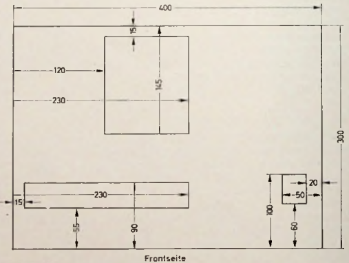
Bild 15. Maßskizze des Deckbleches
