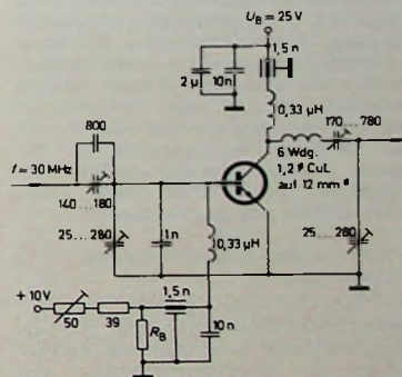
Bild 9. 30-MHz-Einseitenband-Meßschaltung
