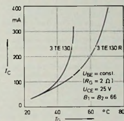
Bild 8. Vergleich der Ruhestromstabilität zwischen emittterwiderstandstabilisiertem und nichtstabilisiertem Transistor gleicher Stromverstärkung B
