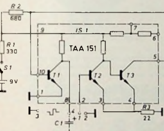
Bild 1. Schaltung des Schmitt-Triggers
