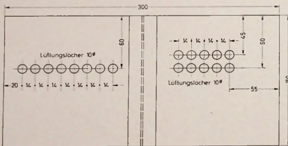
Bild 13. Maßskizze der linken Gehäusesseite
