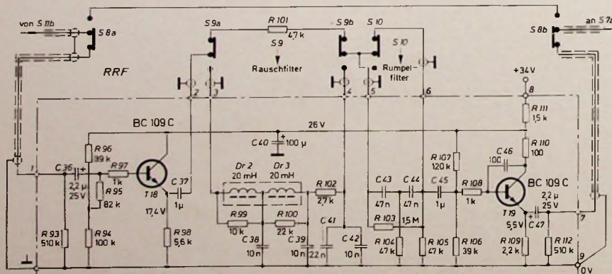
Bild 7. Schaltung der Baugruppe Rausch-Rumpel-Filter (RRF)
