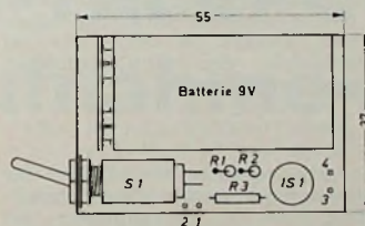
Bild 3. Einzelteilanordnung auf der Montageplatte
