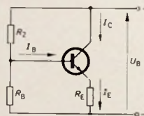
Bild 4. Transistor in Emittter-schaltung; Kollektorruhestrom durch Basisvorspannteiler und Emittterwiderstand stabilisiert
