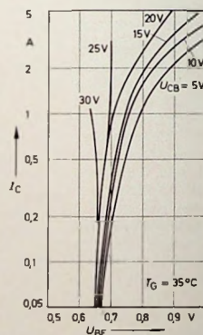
Bild 6. Gemessene I_C - U_{BE} -Kennlinien eines emittterwiderstandstabilisierten Transistors 2 N 4130
