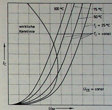
Bild 1. Transistorkennlinien I_C = f(U_{BE})
